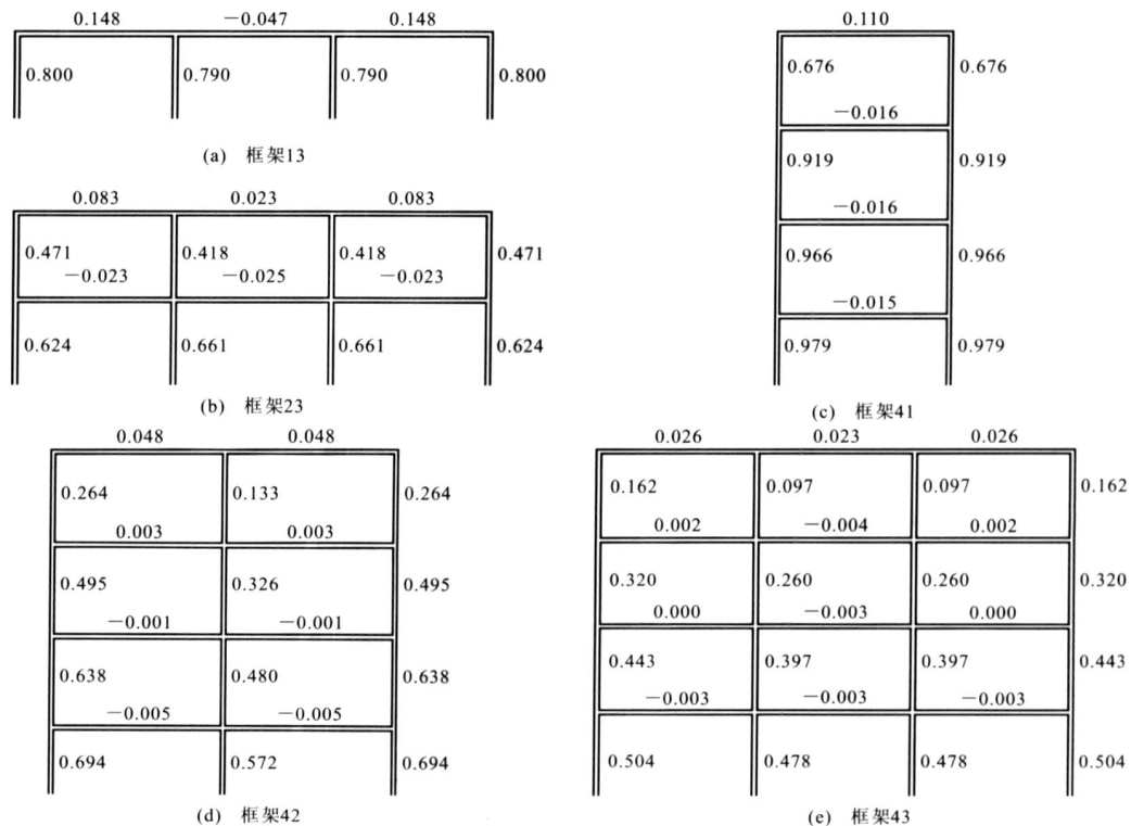
图 2 重力荷载作用下各框架的重要性指标计算结果
